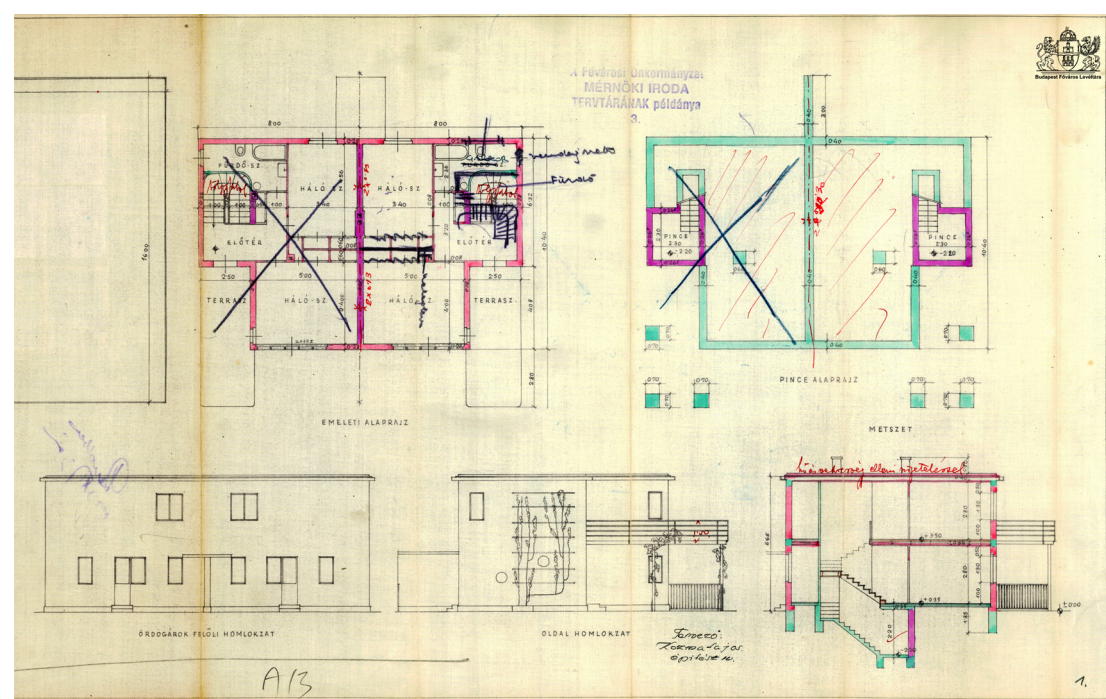
ELSŐ TERVRAJZ, 1930
