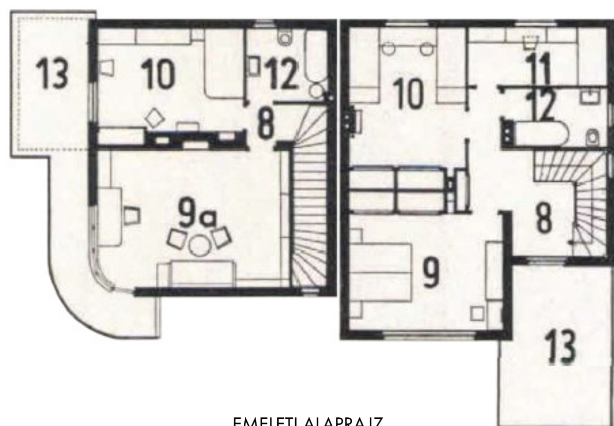
EMELETI ALAPRAJZ
