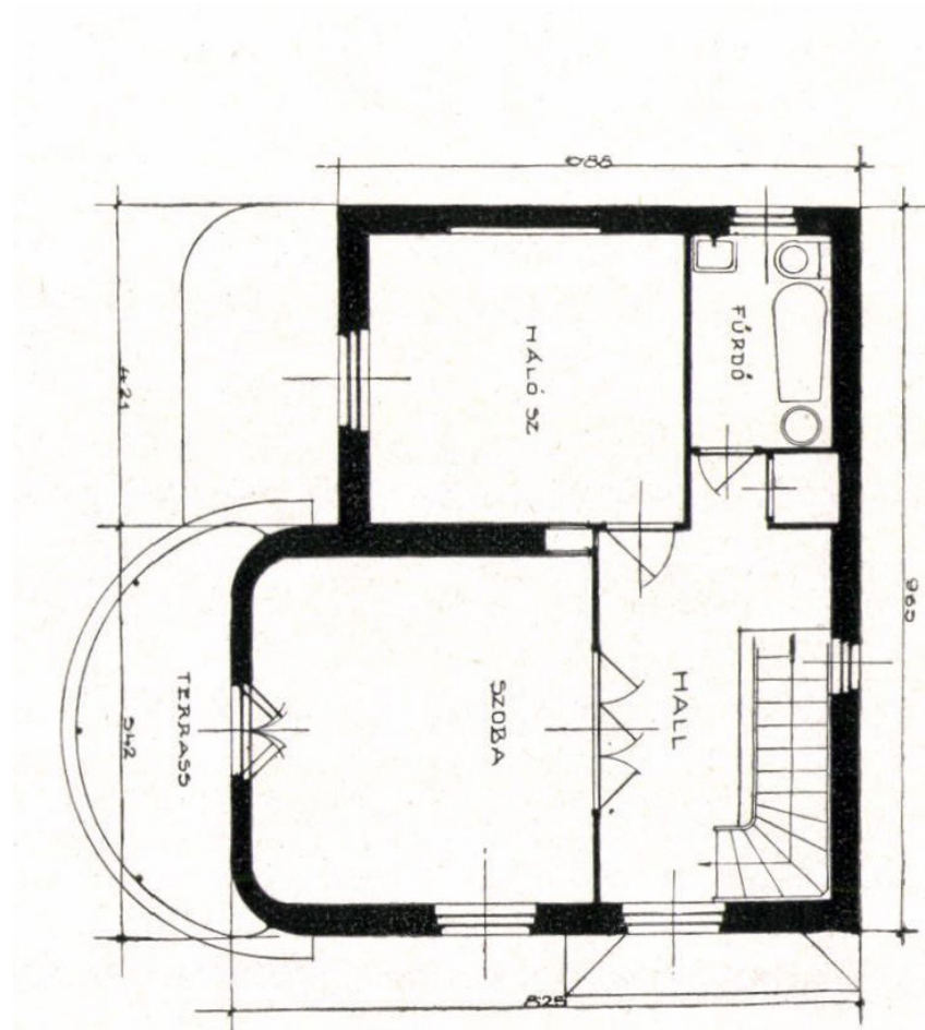
EMELETI ALAPRAJZ
