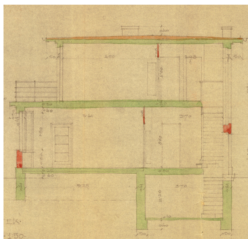
METSZET
