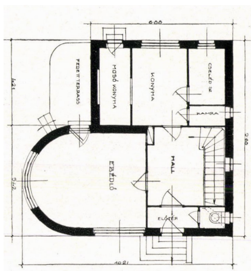
FÖLDSZINTI ALAPRAJZ
