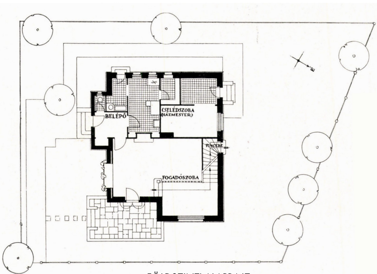
FÖLDSZINTI ALAPRAJZ
