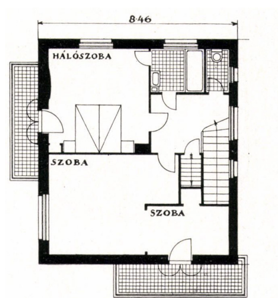
EMELETI ALAPRAJZ
