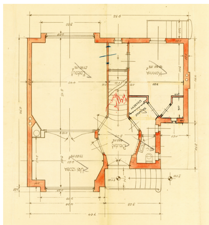
FÖLDSZINTI ALAPRAJZ
