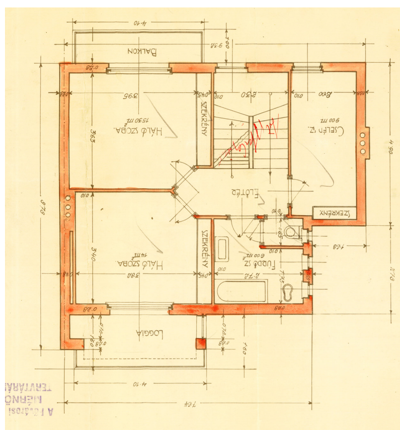
EMELETI ALAPRAJZ
